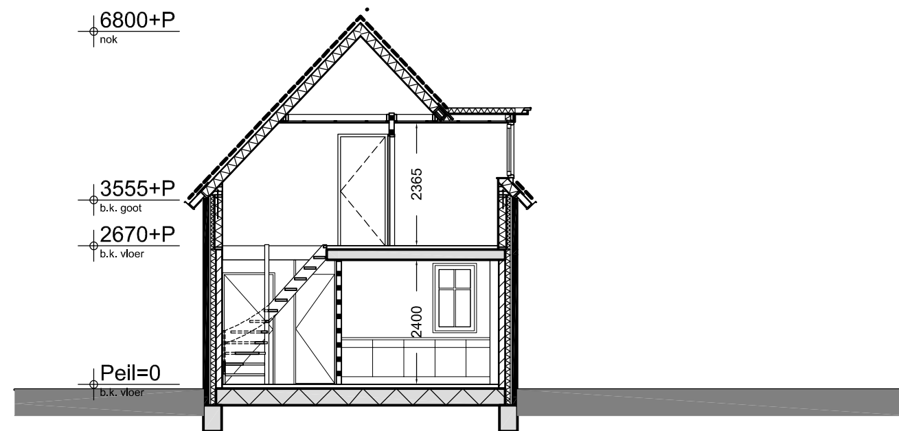
Doorsnede A-A
