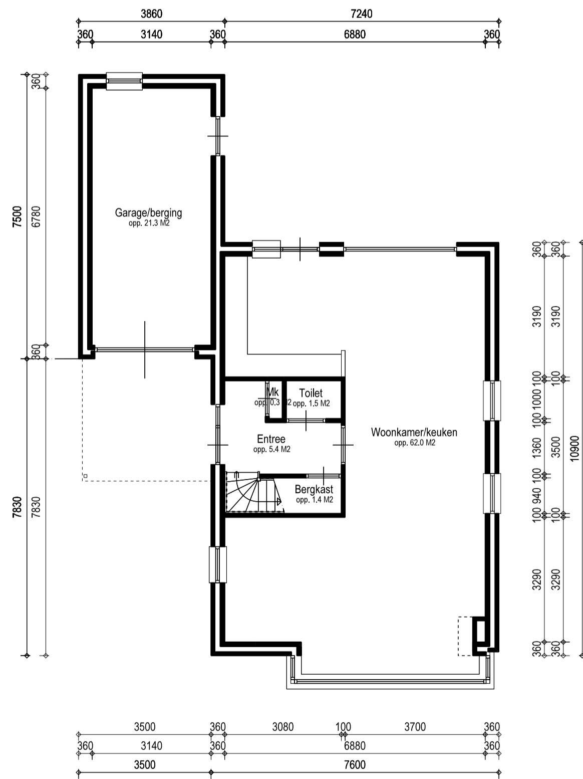
Begane grond
