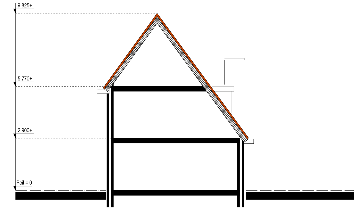
Doorsnede
