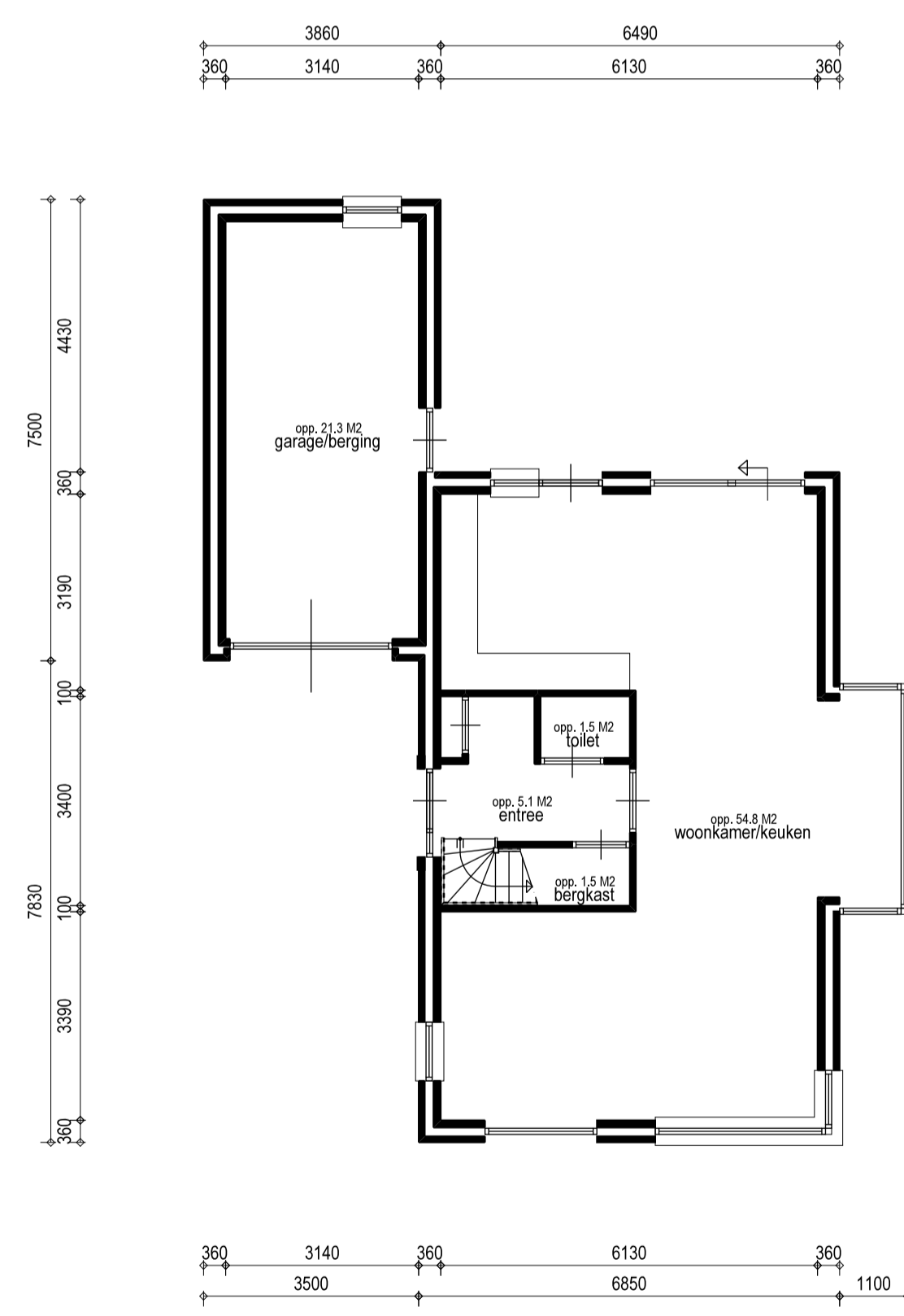
Begane grond
