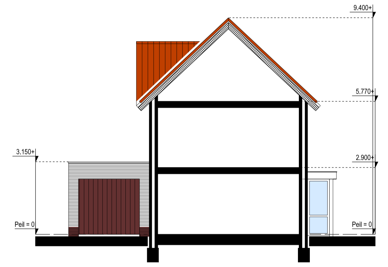
Doorsnede
