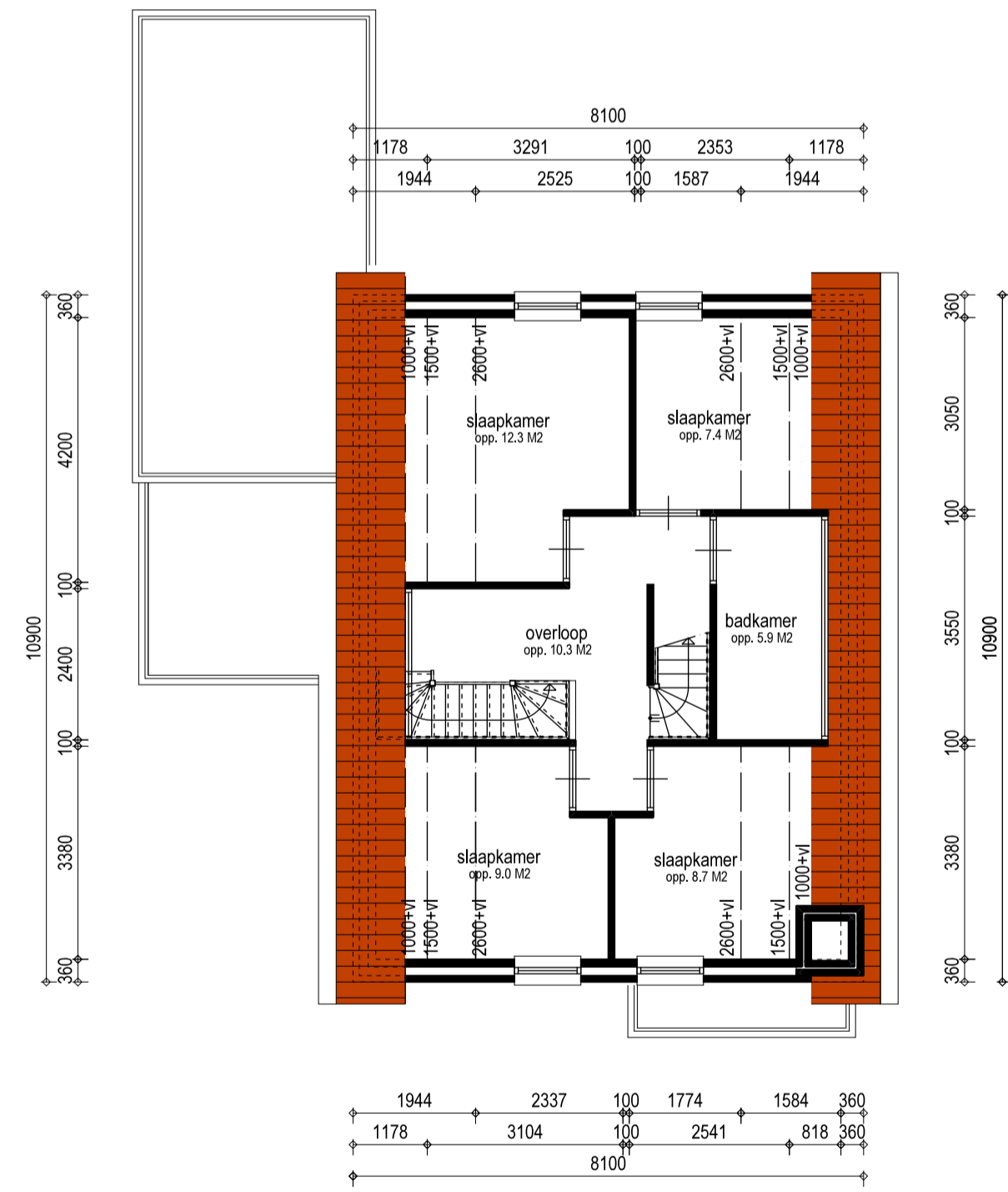
Verdieping
