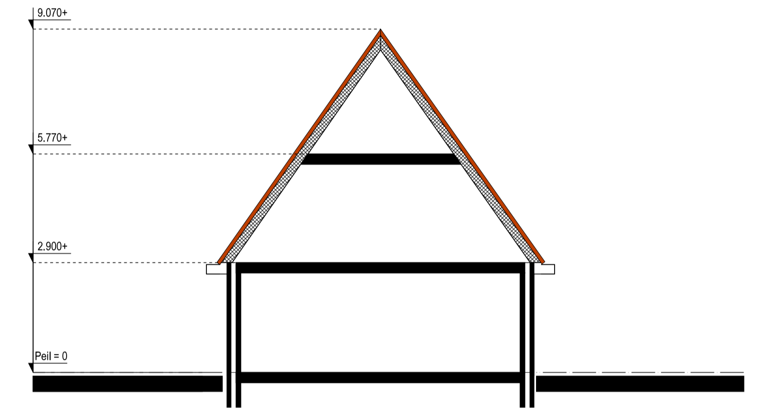
Doorsnede
