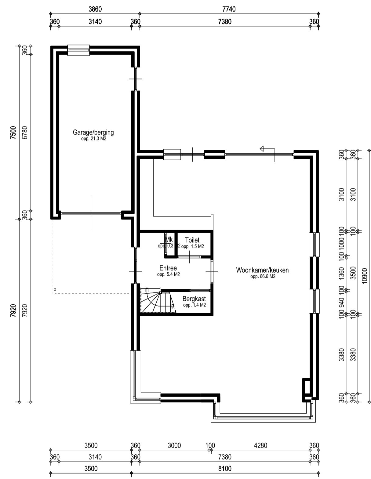
Begane grond
