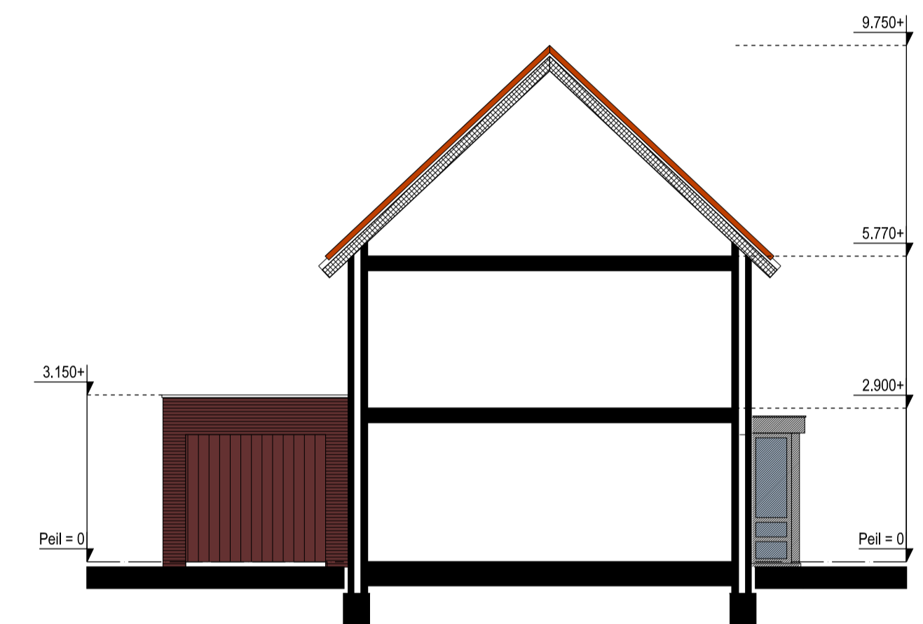
Doorsnede
