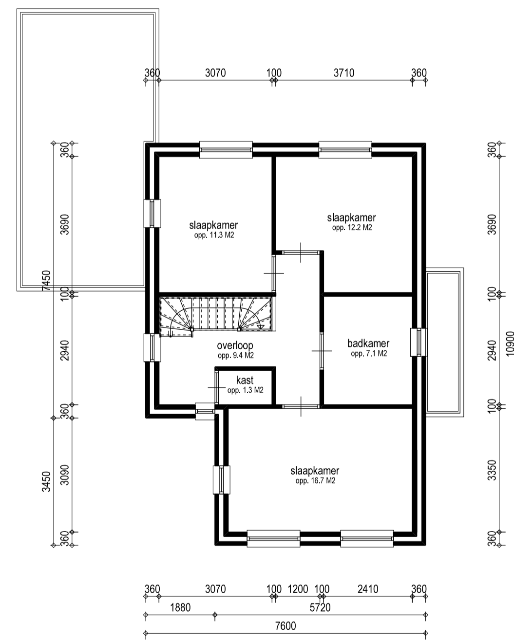
Verdieping
