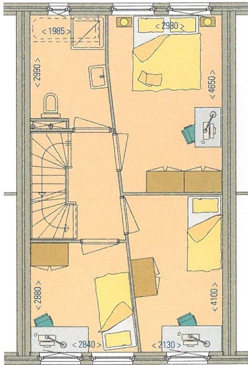
eerste verdieping
