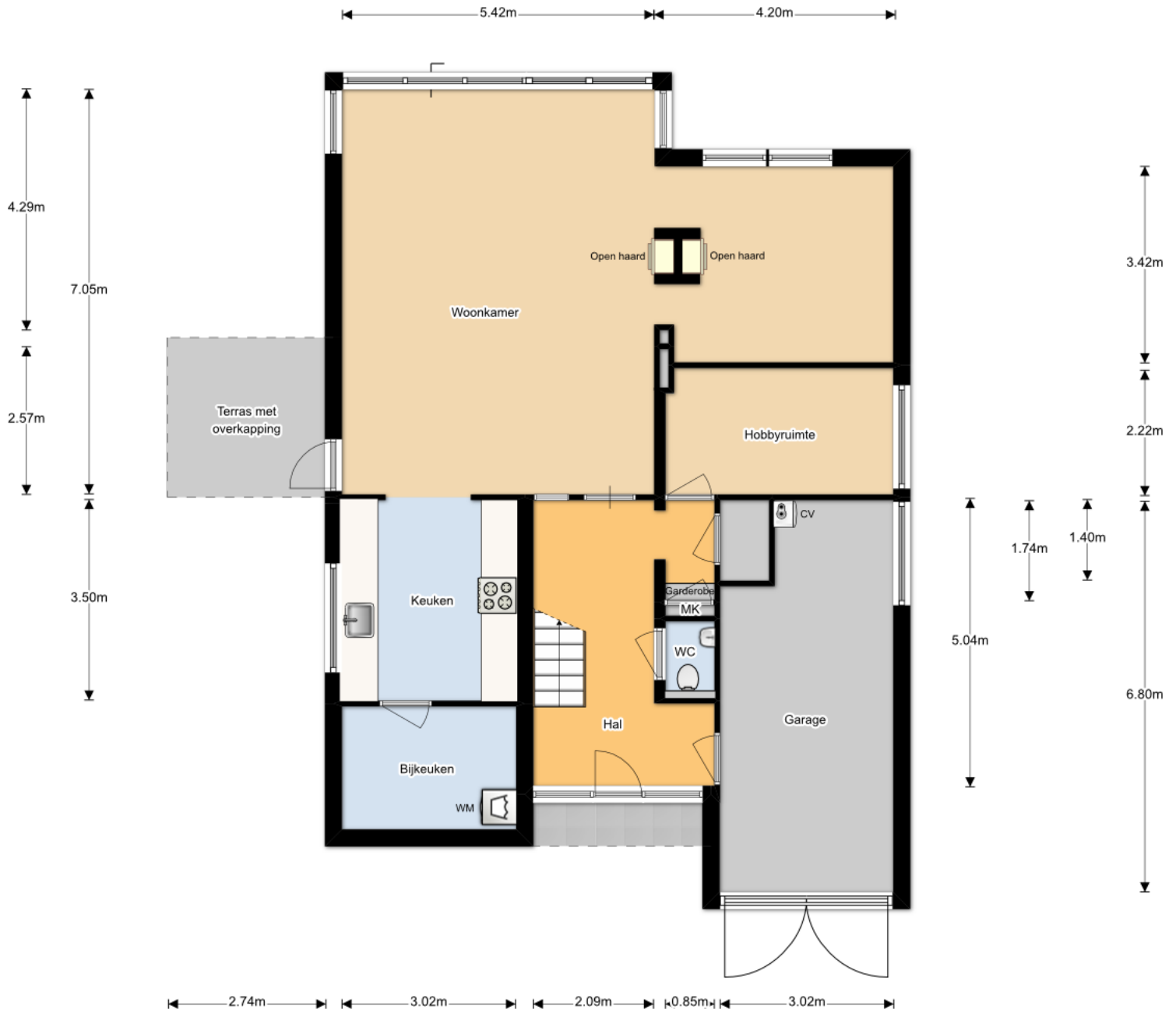
Begane Grond
