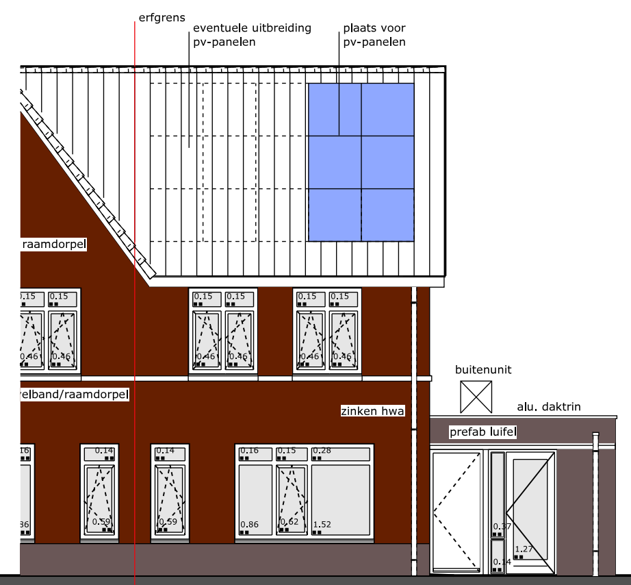
voorgevel
