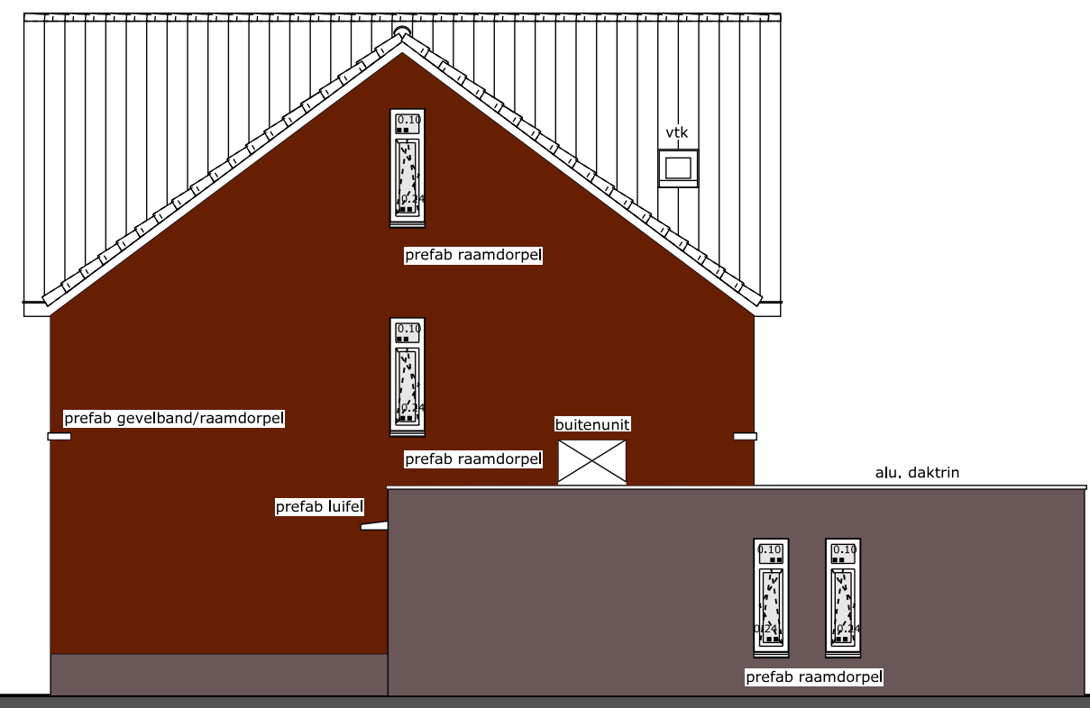
recht zijgevel
