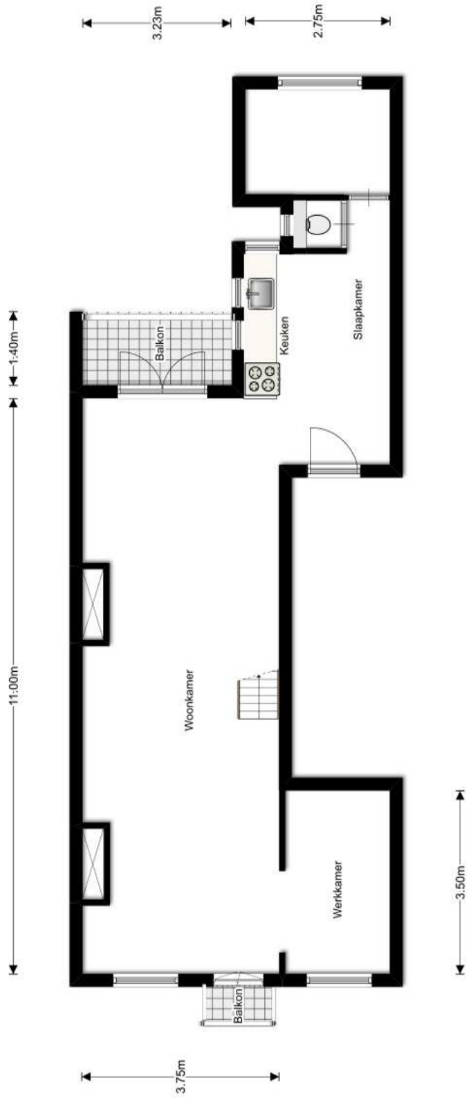
Plattegrond 1
