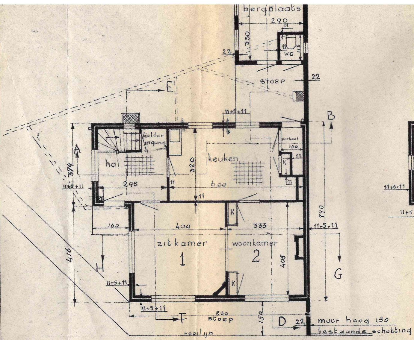
GRONDPLAN
