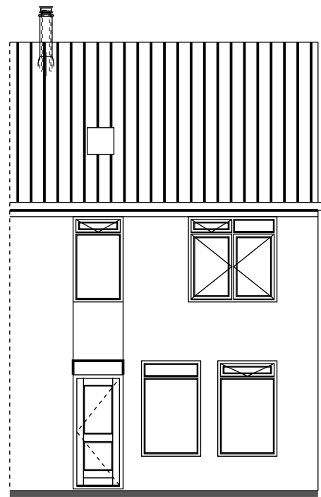
VOORGEVEL
