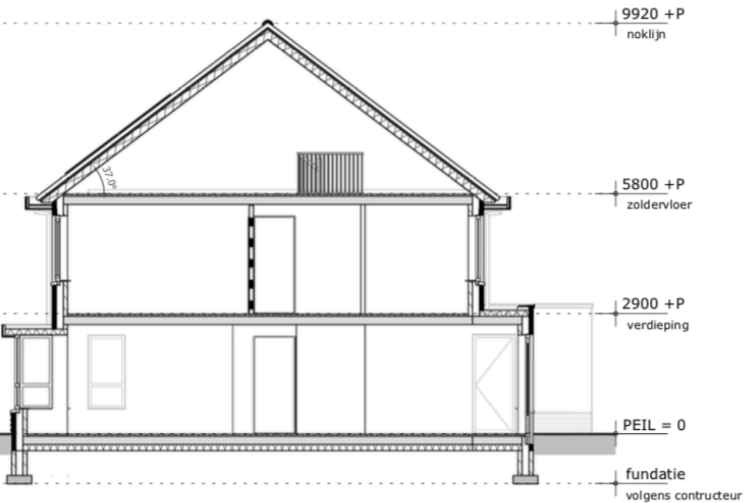
doorsnede B-B
