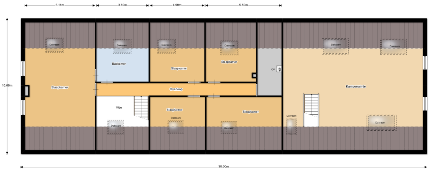
1e Verdieping
