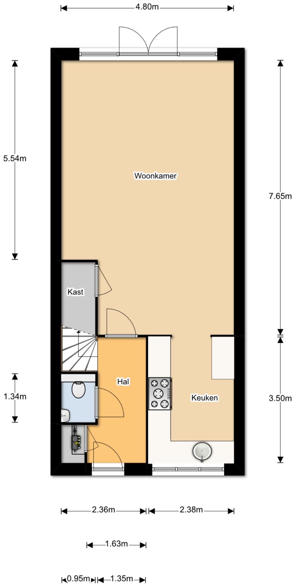
Begane Grond
