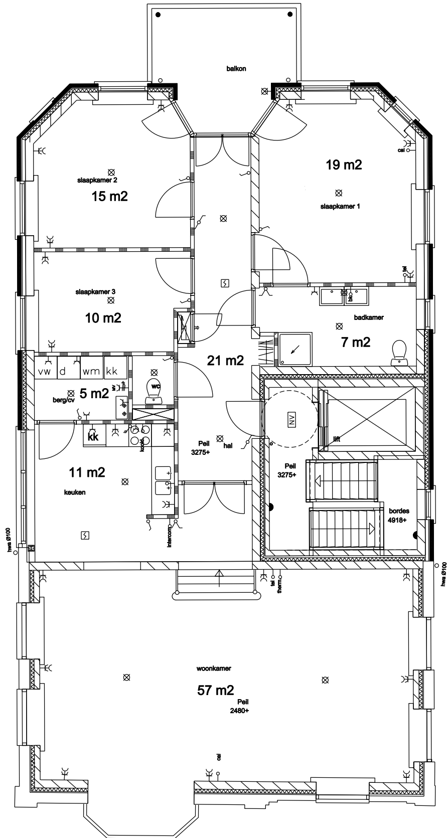
Wierdensestraat 8 Plattegrond 1e verdieping 3275+P
