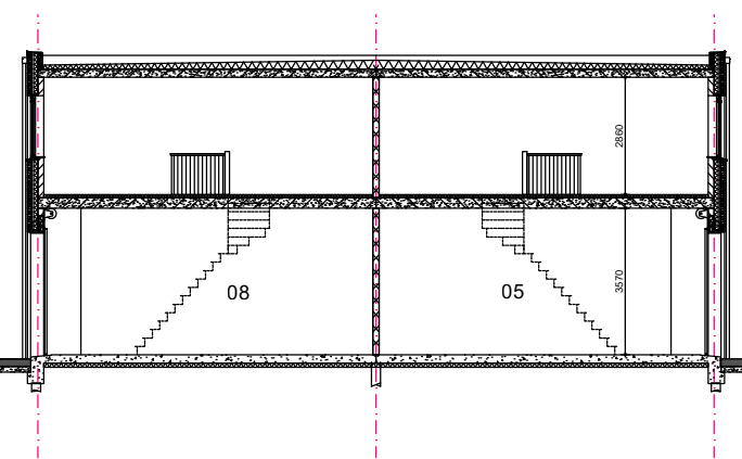
DWARSDOORSNEDE
