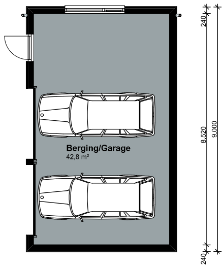
BEGANE GROND
