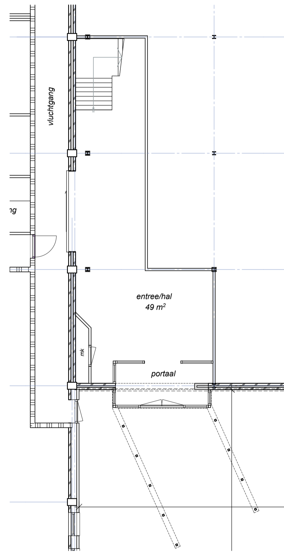
begane grond
